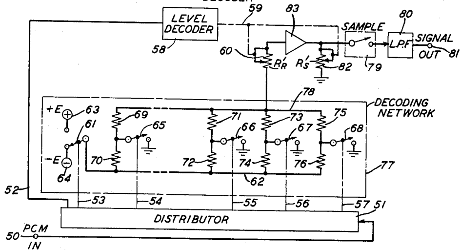
FIG. 2 DECODER
